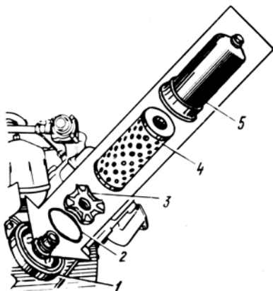
Рис. 68. Масляный фильтр:
