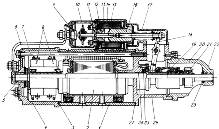
Рис. 51. Стартер:
