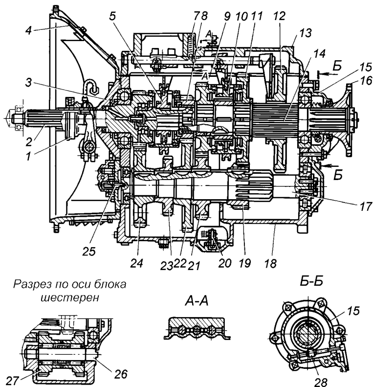
Рис. 119. Коробка передач ЯМЗ-236П:
