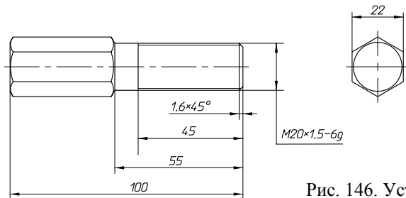
Рис. 146. Установочный винт
