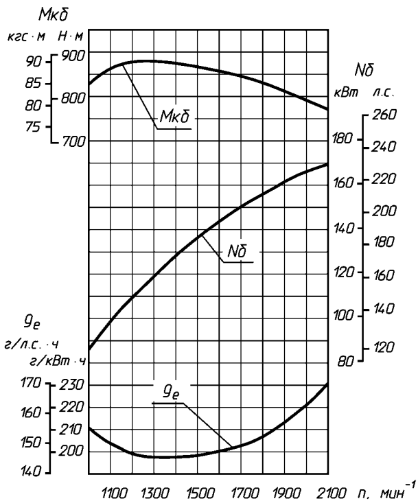
Рис. 3. Скоростная характеристика двигателя ЯМЗ-236НЕ2: M_{кб} - крутящий момент брутто; N_{б} - номинальная мощность брутто; g_e - удельный расход топлива; n - частота вращения коленчатого вала.
