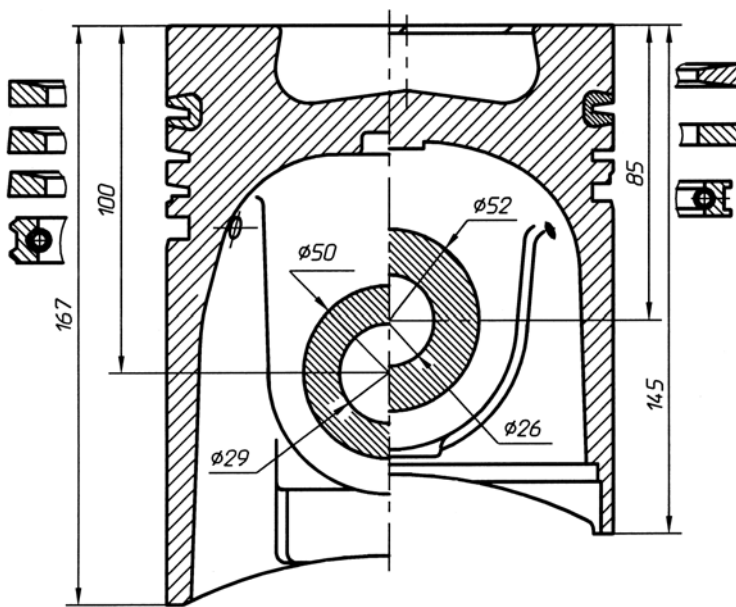
Рис. 18. Поршень, поршневые кольца, палец:
