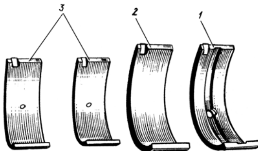
Рис. 16. Вкладыши подшипников коленчатого вала:
