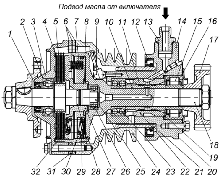
Рис. 43. Привод вентилятора
