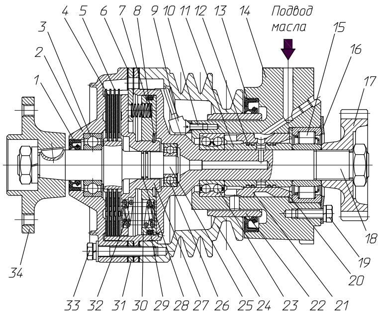
Рис. 123. Привод вентилятора
