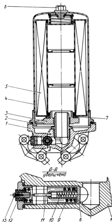
Рис. 22. Масляный фильтр: 1–корпус фильтра; 2–прокладка колпака; 3–замковая крышка; 4–колпак фильтра; 5–фильтрующий элемент; 6–головка колпака; 7–прокладка фильтрующего элемента; 8–плунжер клапана; 9–пружина клапана; 10–пружина сигнализатора; 11–подвижный контакт сигнализатора; 12–неподвижный контакт; 13–клемма
